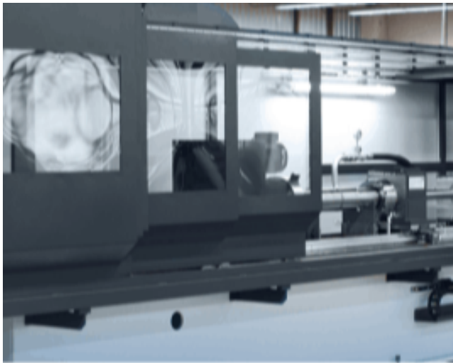
TIBO, Tiefbohrtechnik für Rundteile • 1, 2, 3, 4, 6 or 12 Spindel-Ausführung • Bohr-Ø: 2-40 mm; Bohrtiefe bis zu 4.500 mm „The first choice for deep hole drilling. Worldwide.“
